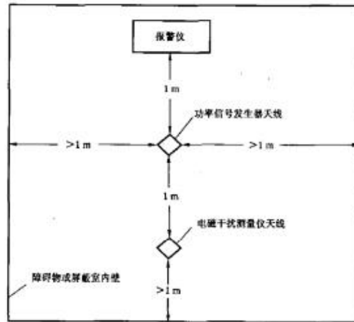
图2 天线位置图
