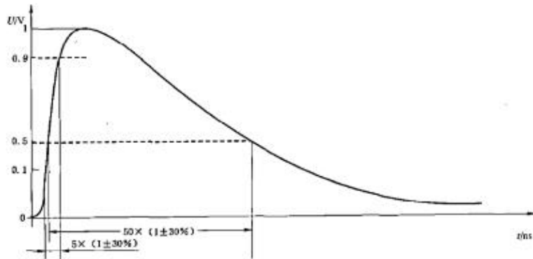
图3 50Ω负载时单脉冲波形
